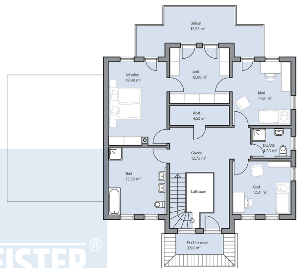
Haus Dalmann Grundriss
