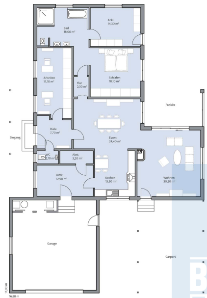
Haus Dittmer Grundriss
